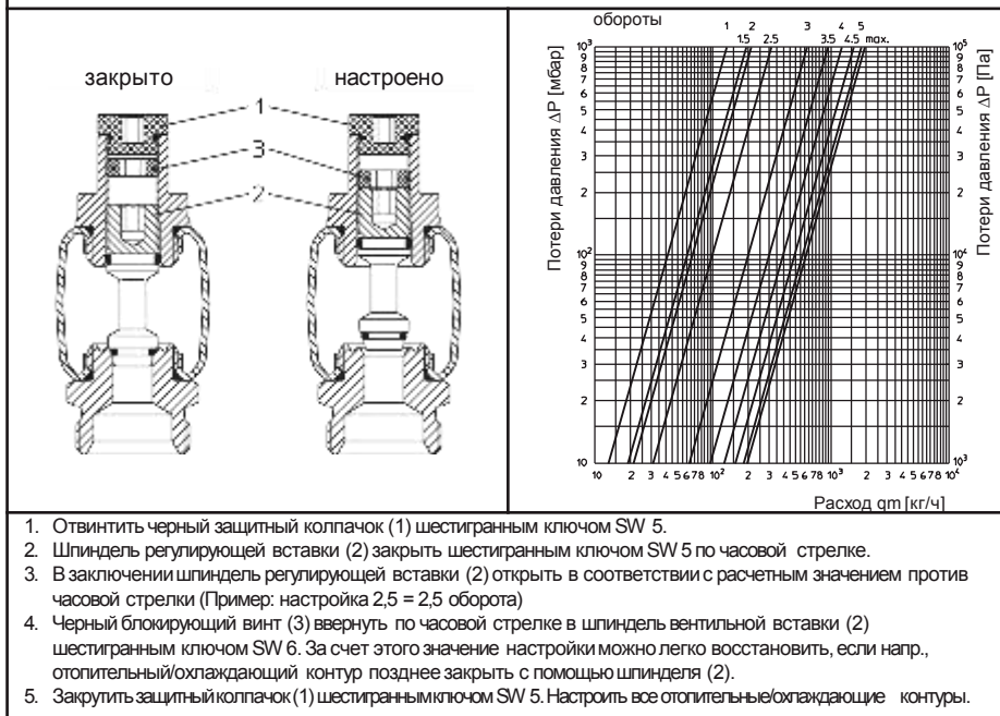
Рис. 7.3 Настройка регулирующих вставок
