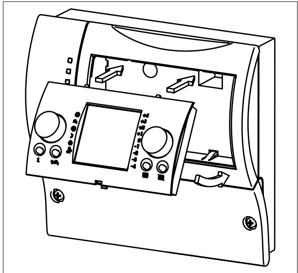
Рис. 4.10 Установка модуля управления BM в модуль расширения
