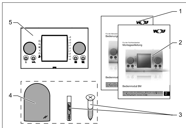
Рис. 4.1 Объем поставки модуля управления VM с датчиком наружной температуры/без датчика
