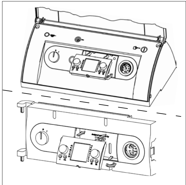
Рис. 4.9 Установить модуль управления VM
