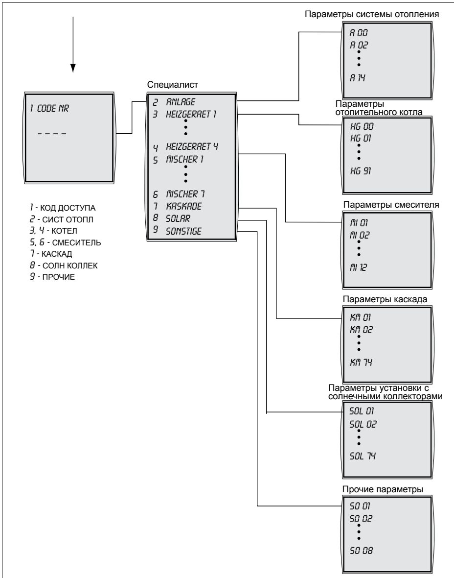
Рис. 5.3 Структура меню модуля управления ВМ
