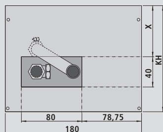
Торцевая сторона
