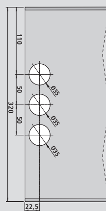
Вид сверху
