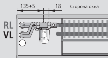
Вид сверху
