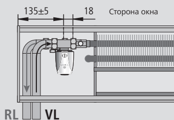
Вид сверху
