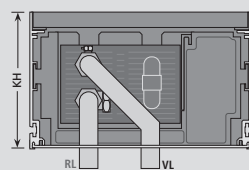
Сечения
