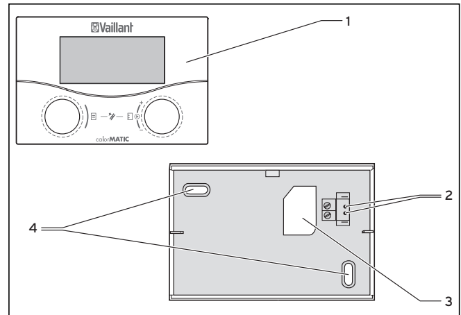
Рис. 4.4 Монтаж в качестве прибора дистанционного управления
